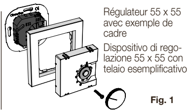
Régulateur 50 x 50 avec exemple de cadre et cadre intermédiaire Dispositivo di regolazione 50 x 50 con telaio esemplificativo e telaio intermedio
